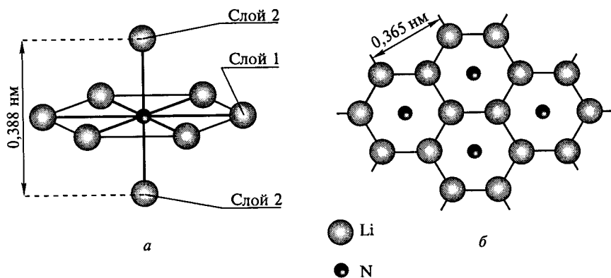
Рис. 2.4. Структура кристаллического нитрида лития:
