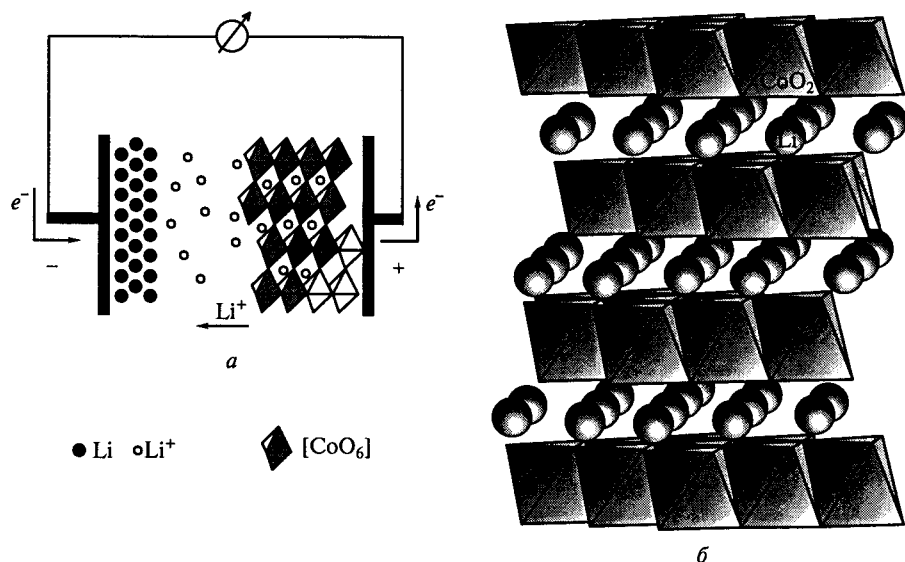
Рис. 2.2. Схема работы литиевого элемента при разрядке (а); строение кристалла кобальтита лития (б) (ионы лития расположены между слоями, образованными октаэдрами CoO_6 )
