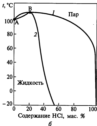
Рис. 8.10. Фазовое равновесие жидкость — пар в системе НF—Н 2 О (а) и НСl—Н 2 О (б) при P = 1 атм
