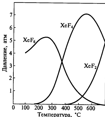
Рис. 9.2. Зависимость равновесного давления ди-, тетра- и гексафторида ксенона от температуры
