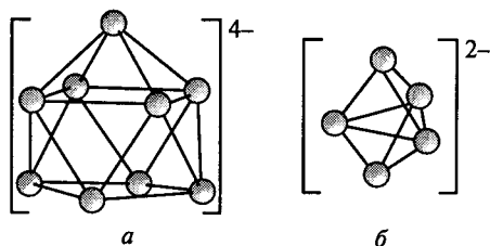
Рис. 5.14. Структура ионов Цинтля:
