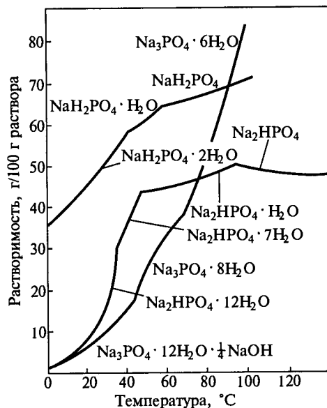
Рис. 6.27. Зависимость растворимости фосфатов натрия от температуры
