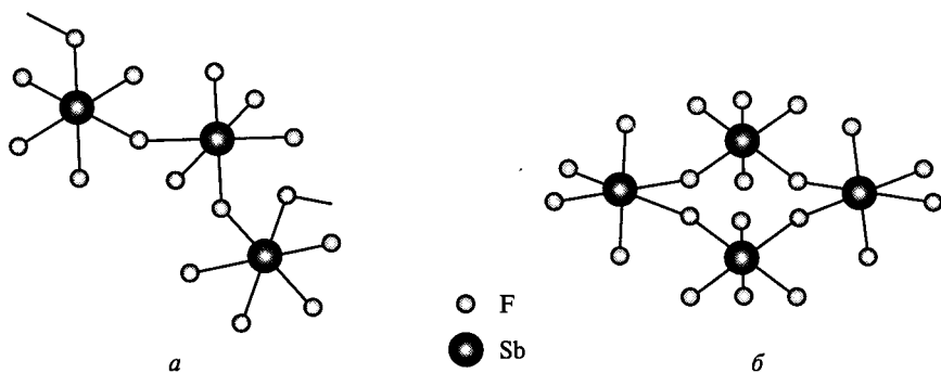
Рис. 6.30. Строение молекулы \text{SbF}_5 в жидком (а) и твердом (б) состоянии
