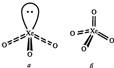
Рис. 9.7. Строение молекул \text{XeO}_3 (а) и \text{XeO}_4 (б)
