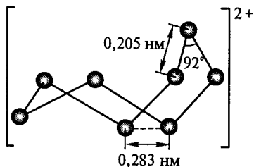
Рис. 7.10. Строение катиона \text{S}_8^{2+} в структуре [\text{S}_8]^{2+}[\text{AsF}_6]_2^-
