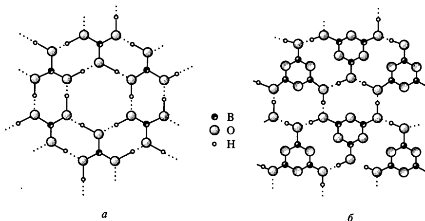
Рис. 4.9. Части слоя ортоборной B(OH)_3 (а) и метаборной HBO_2 (б) кислоты (сплошными линиями показаны ковалентные связи, пунктирными линиями — водородные связи)
