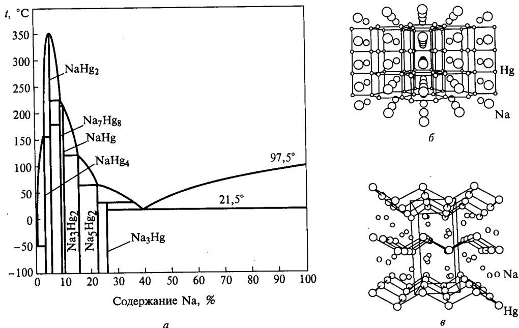
Рис. 2.5. Диаграмма состояния системы \text{Na} - \text{Hg} ( a ); схема упаковки атомов натрия и ртути в структуре \text{NaHg}_2 ( б ) и \text{NaHg} ( е )
