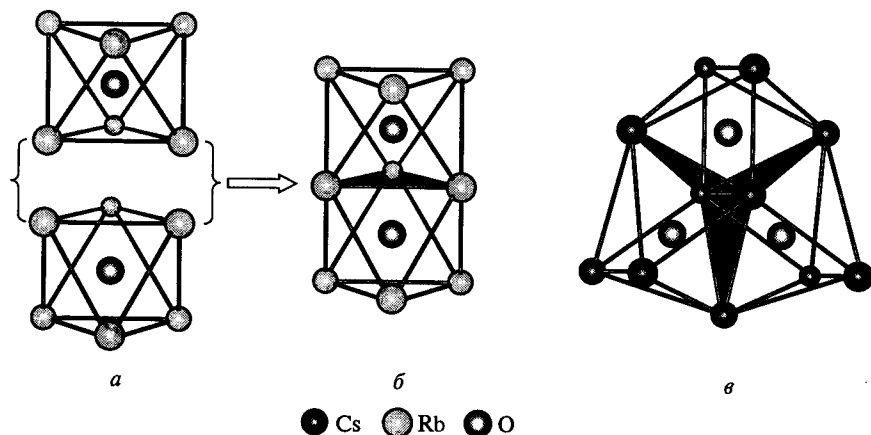
Рис. 2.7. Структуры субоксидов: а — \text{RbO}_6 ; б — \text{Rb}_9\text{O}_2 ; в — \text{Cs}_{11}\text{O}_3
