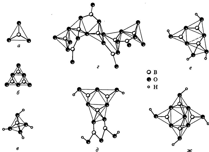
Рис. 4.10. Строение борат-анионов:
