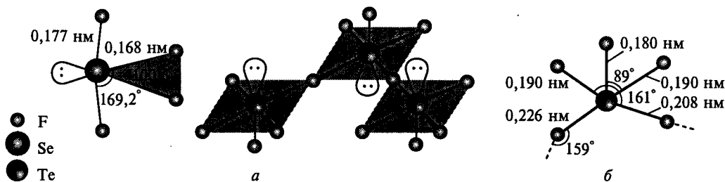
Рис. 7.25. Строение молекул: a — \text{SeF}_4 в газовой фазе; б — твердого \text{TeF}_4
