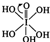
\text{H}_5\text{IO}_6
