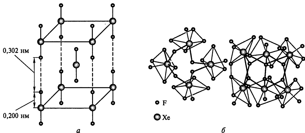
Рис. 9.4. Строение:
