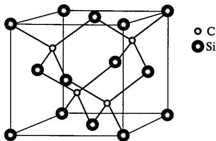
Рис. 5.13. Структура карборунда
