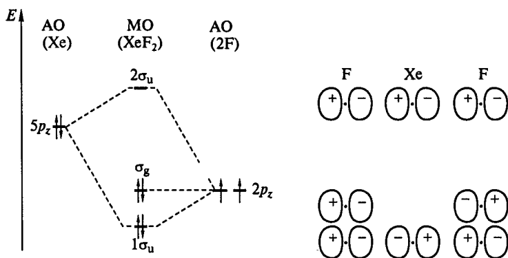
Рис. 9.5. Схема молекулярных орбиталей молекулы \text{XeF}_2 . Справа показаны комбинации атомных орбиталей, участвующих в формировании каждой из молекулярных орбиталей молекулы
