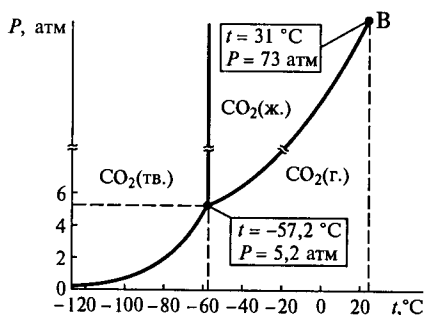
Рис. 5.18. Фазовая диаграмма CO 2
