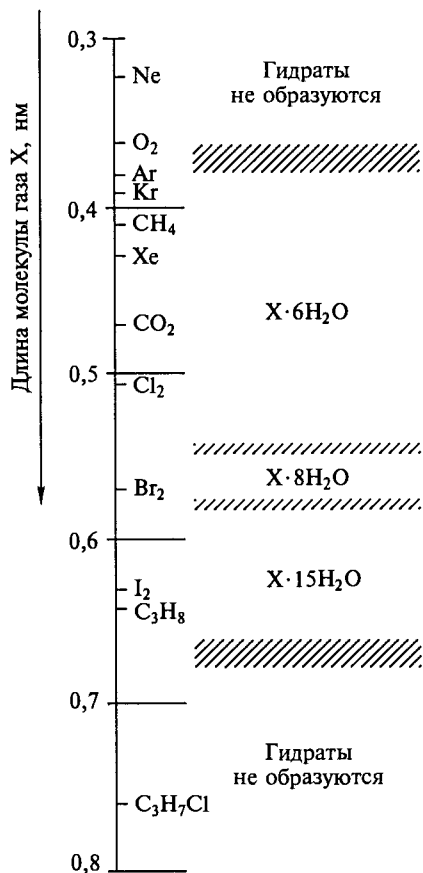
Рис. 1.17. Образование гидратов в зависимости от размера молекул газа
