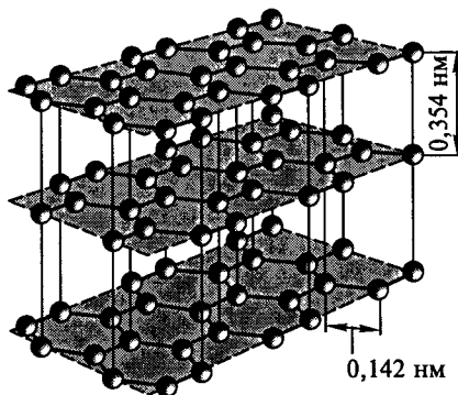
Рис. 5.4. Строение графита
