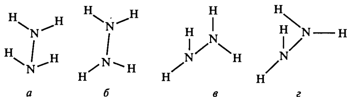
Рис. 6.14. Цис- (а), транс- (б), полужаслоненная- (в), гош- (г) формы (конформеры) гидразина
