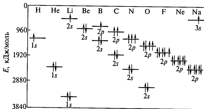
Рис. 3.8. Изменение энергии 1s-, 2s- и 2p-орбиталей у атомов 2-го периода Периодической системы
