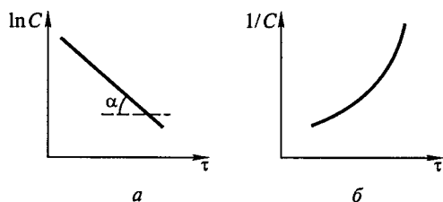
Рис. 2.3. График зависимости C=f(\tau) для реакции разложения H_2O_2 : а — в координатах \ln C-\tau ; б — 1/C-\tau
