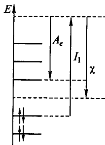
Рис. 3.11. Энергетическая диаграмма, иллюстрирующая связь энергии сродства к электрону ( A_e ) и электроотрицательности ( \chi )
